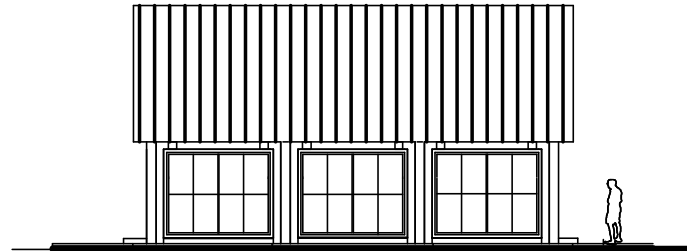
POHLED JIŽNÍ
