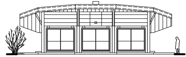
POHLED JIŽNÍ
